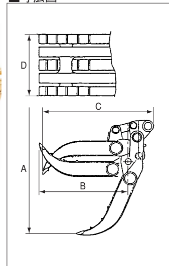
■寸法図
