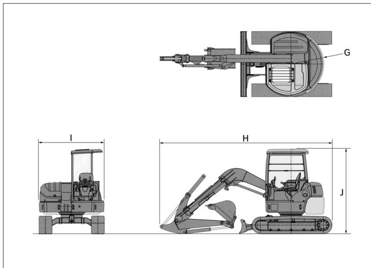
ZAXIS75UR
